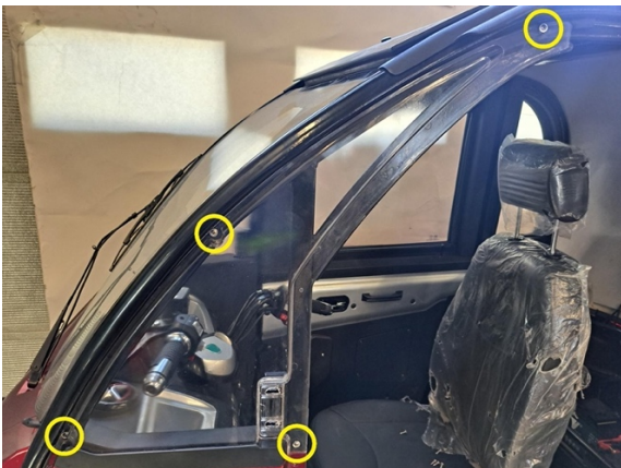
Irrota etummaisena sivuikkunan kiinnitysruuvit. (ristipäämeisseli ph2).
