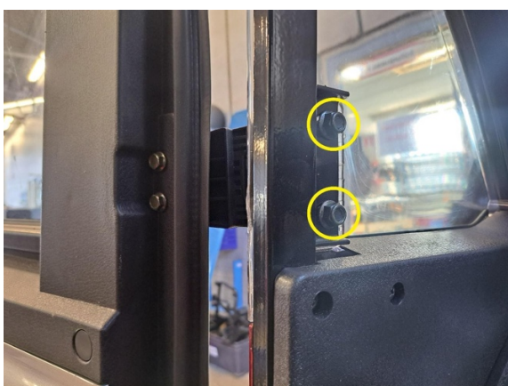
Irrota oven saranoiden kiinnitysmutterit. (hylsy 12 mm).
